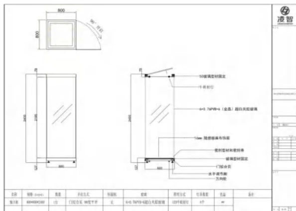
独立柜800*800*2400
