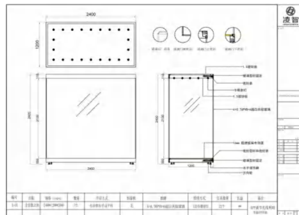
独立柜1200*2400*2400
