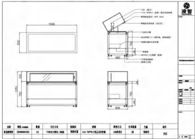
带箱体：1500*600*1050
