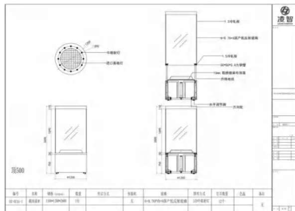
圆形柜1200*2600
