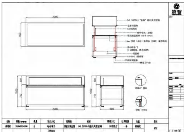
顶升柜：2000*800*1050
