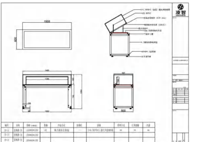
直角柜：1200/1500/1800*600*1050
