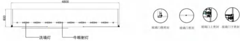
4800*800*3000
