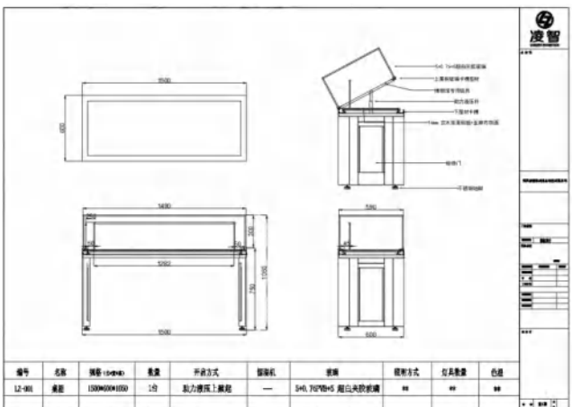
两腿柜：1500*600*1050
